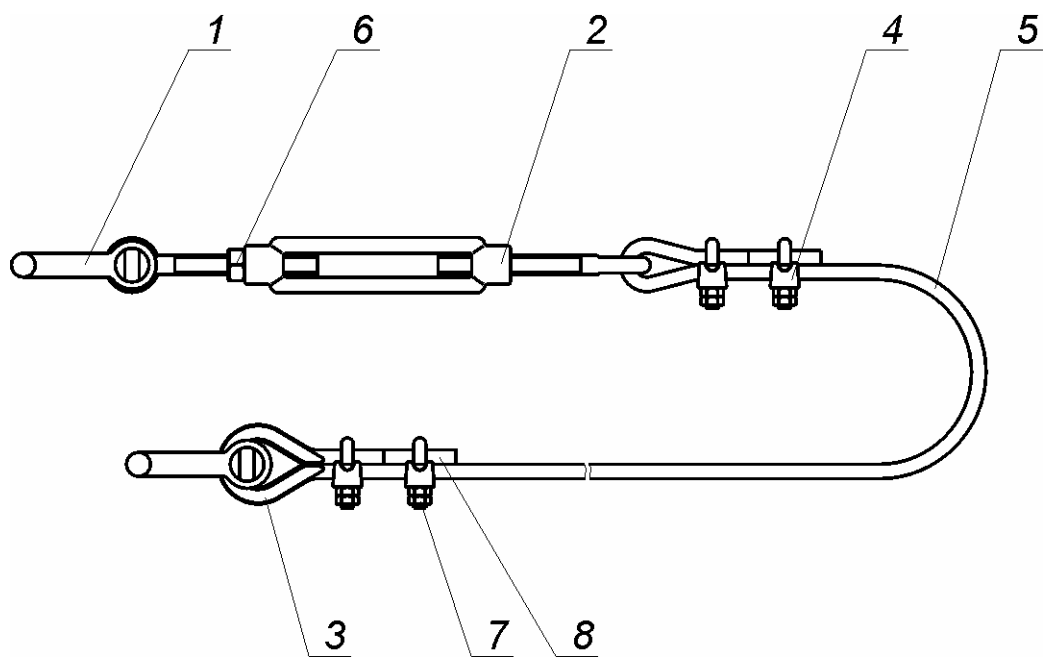
Rys. 40 Linka spinająca
