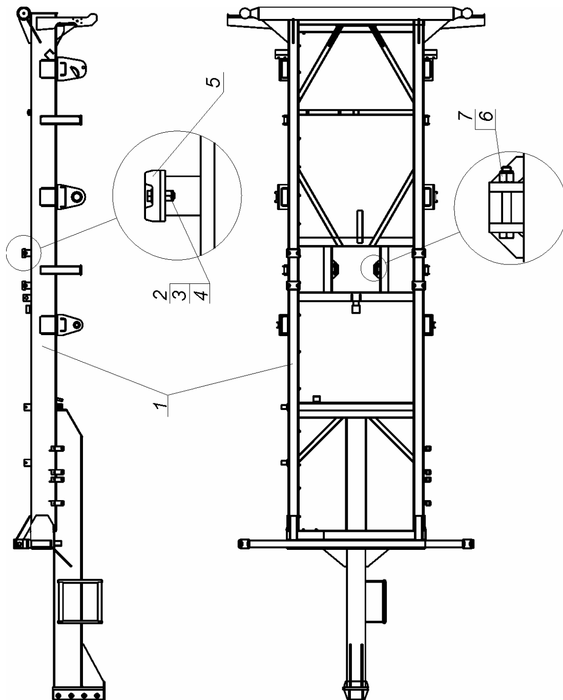
Rys. 20 Rama dolna
