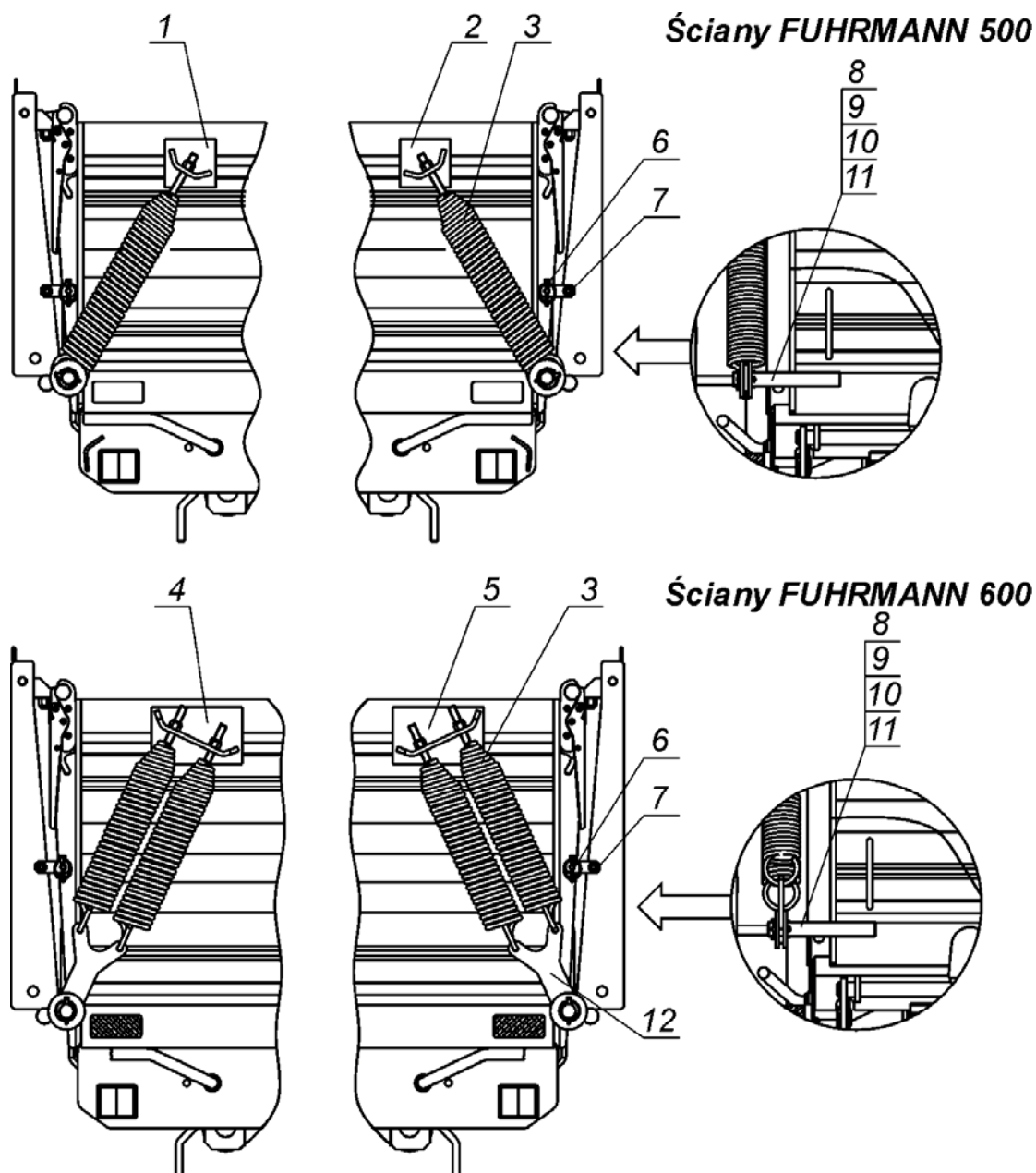
Rys. 44 Mechanizm odciągowy bort
