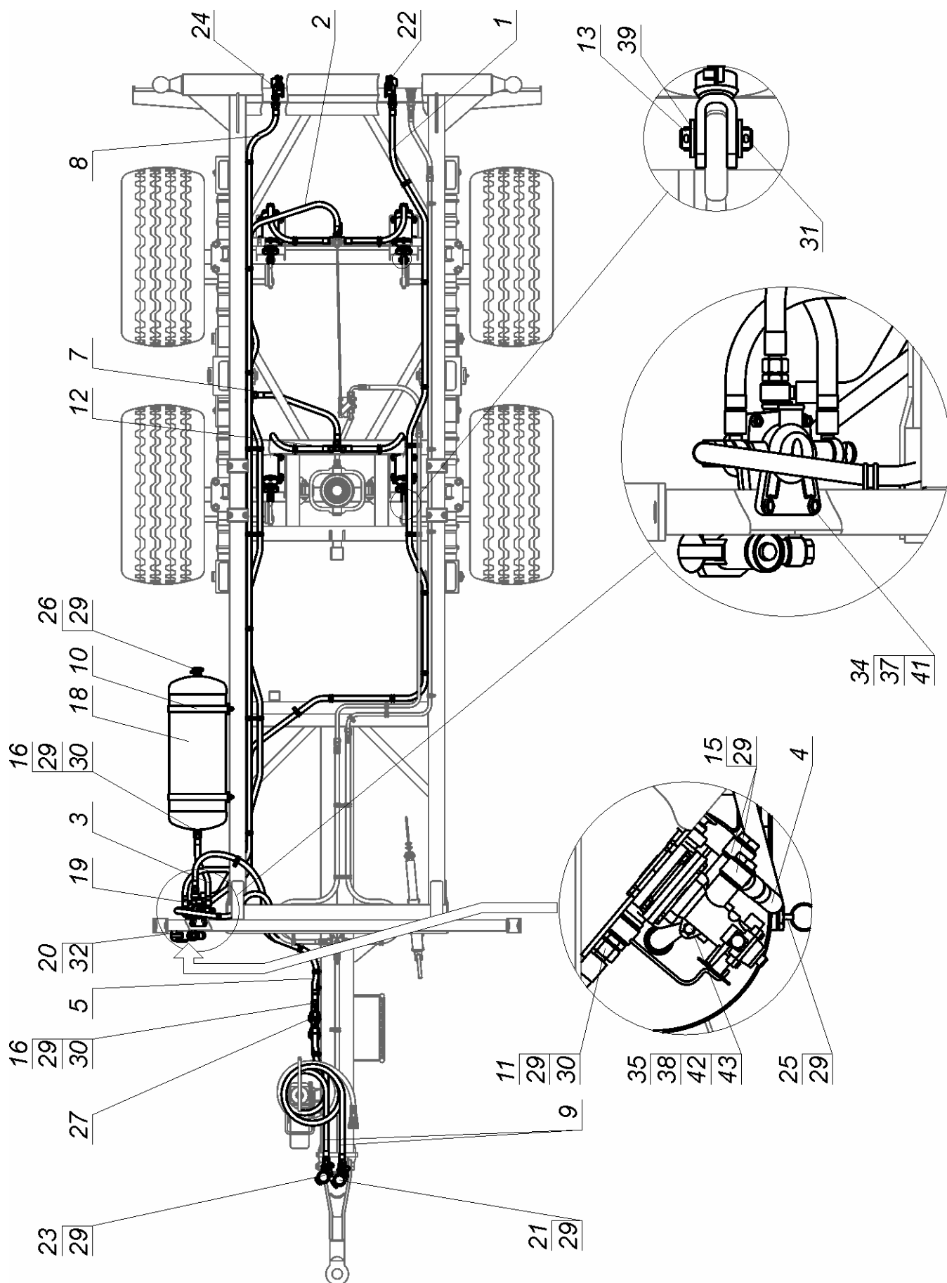
Rys. 25 Instalacja pneumatyczna dwuprzewodowa, widok z góry
