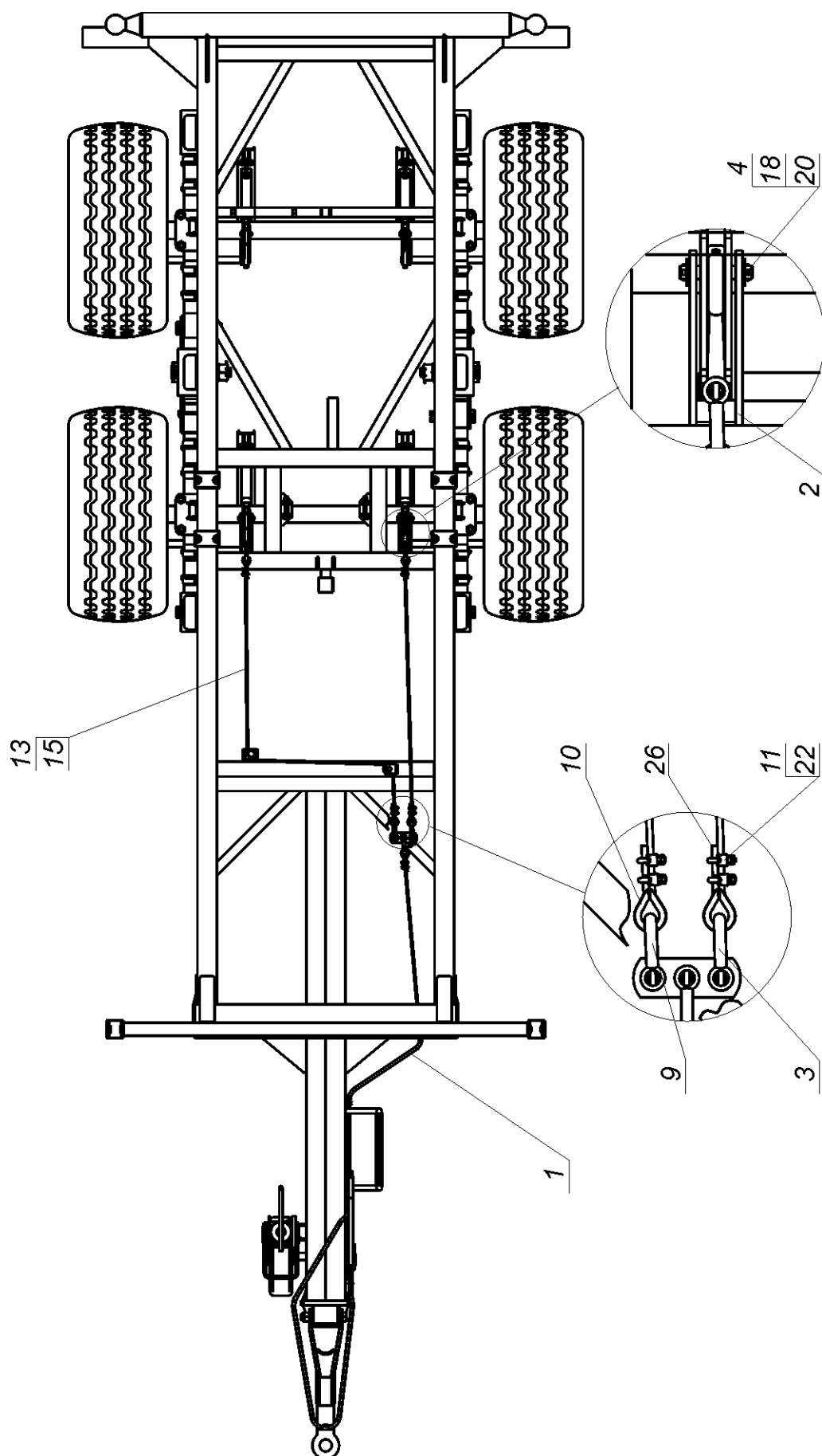
Rys. 29 Hamulec ręczny dźwigniowy, widok z góry
