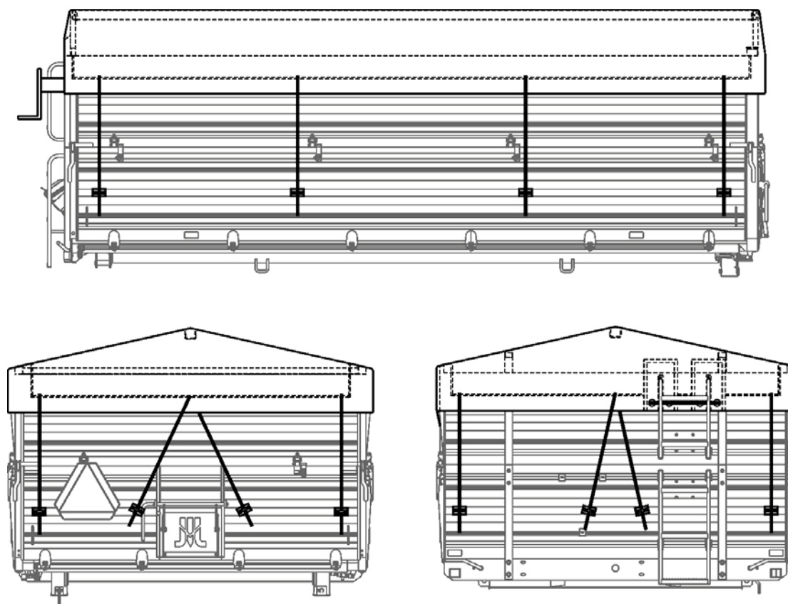
Rys. 51 Widok zamocowania plandeki i stelaża
