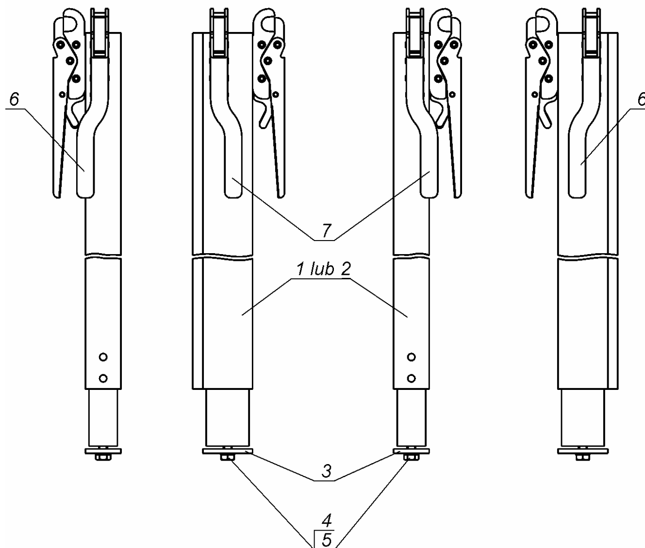
Rys. 53 Słupki
