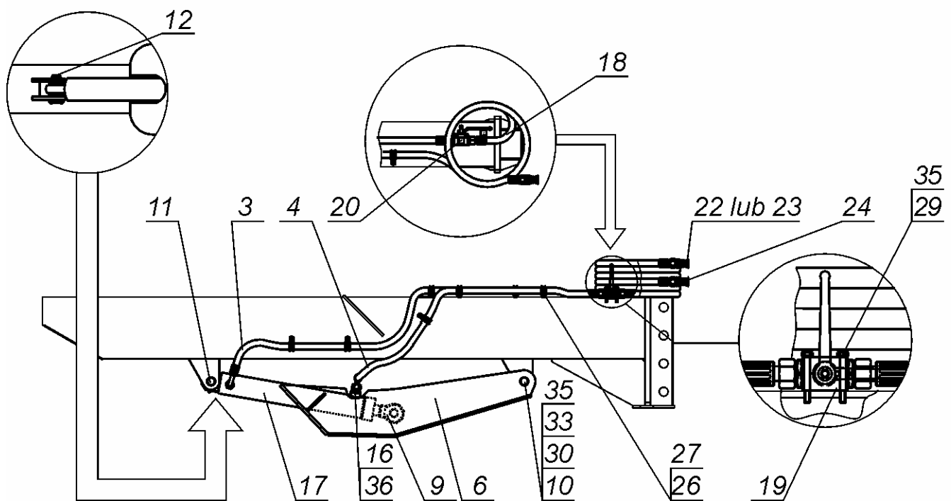
Rys. 33 Podpora hydrauliczna nożycowa
