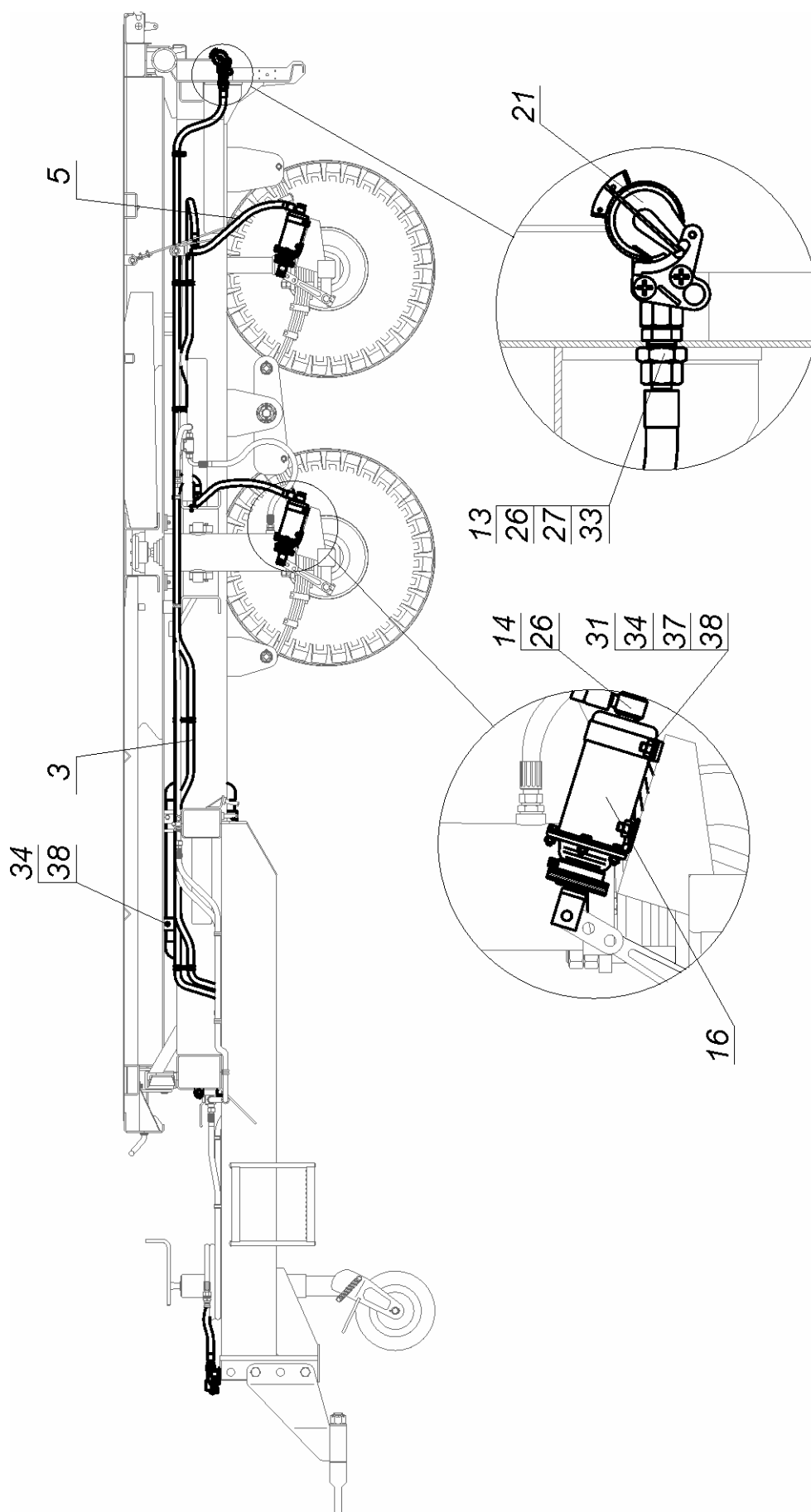
Rys. 22 Instalacja pneumatyczna jedнопроводовая, widok z boku
