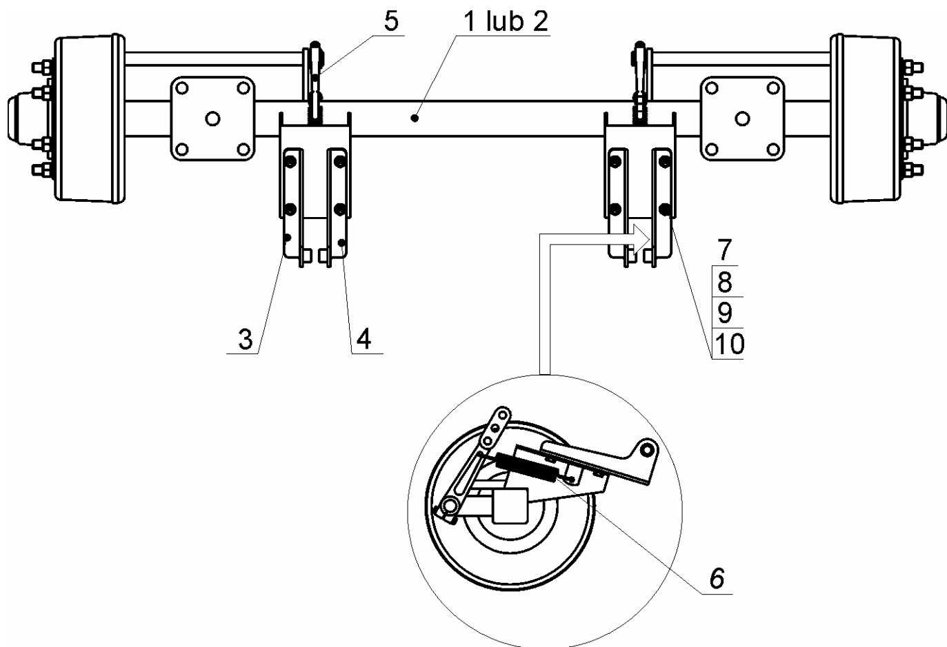
Rys. 39 Oś jezdna
