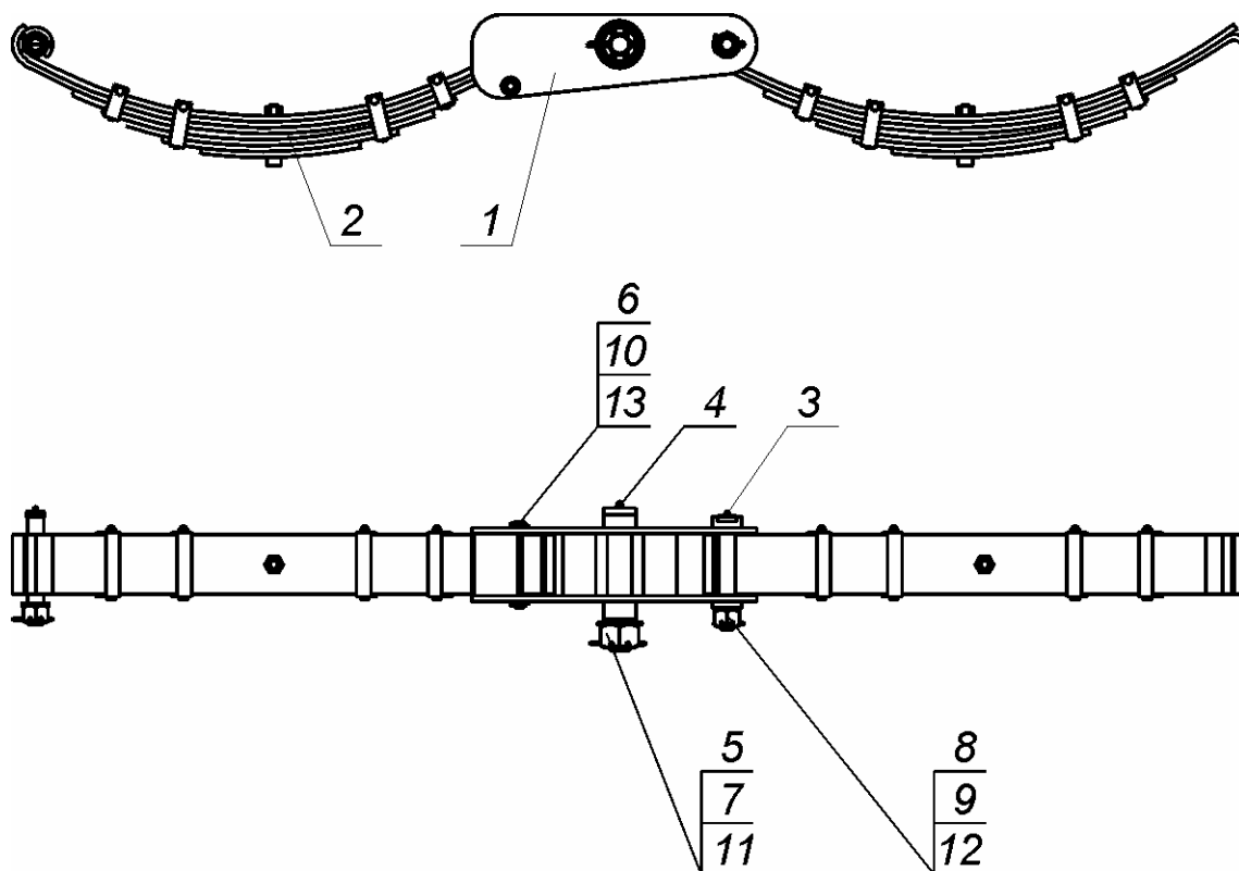
Rys. 42 Zawieszenie resorowe prawe
