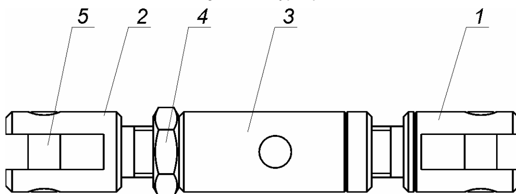
Rys. 47 Ciężno, kpl.
