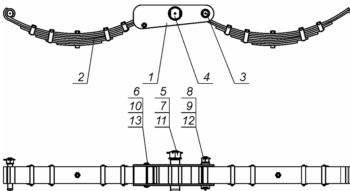
Rys. 43 Zawieszenie resorowe lewe
