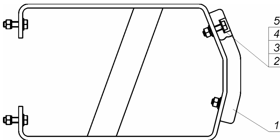
Rys. 48 Odbojnik ściany tylnej
