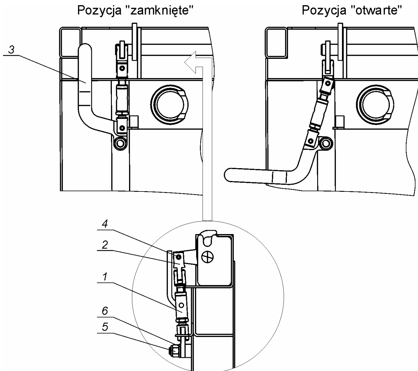
Rys. 45 Zamknięcie tylne
