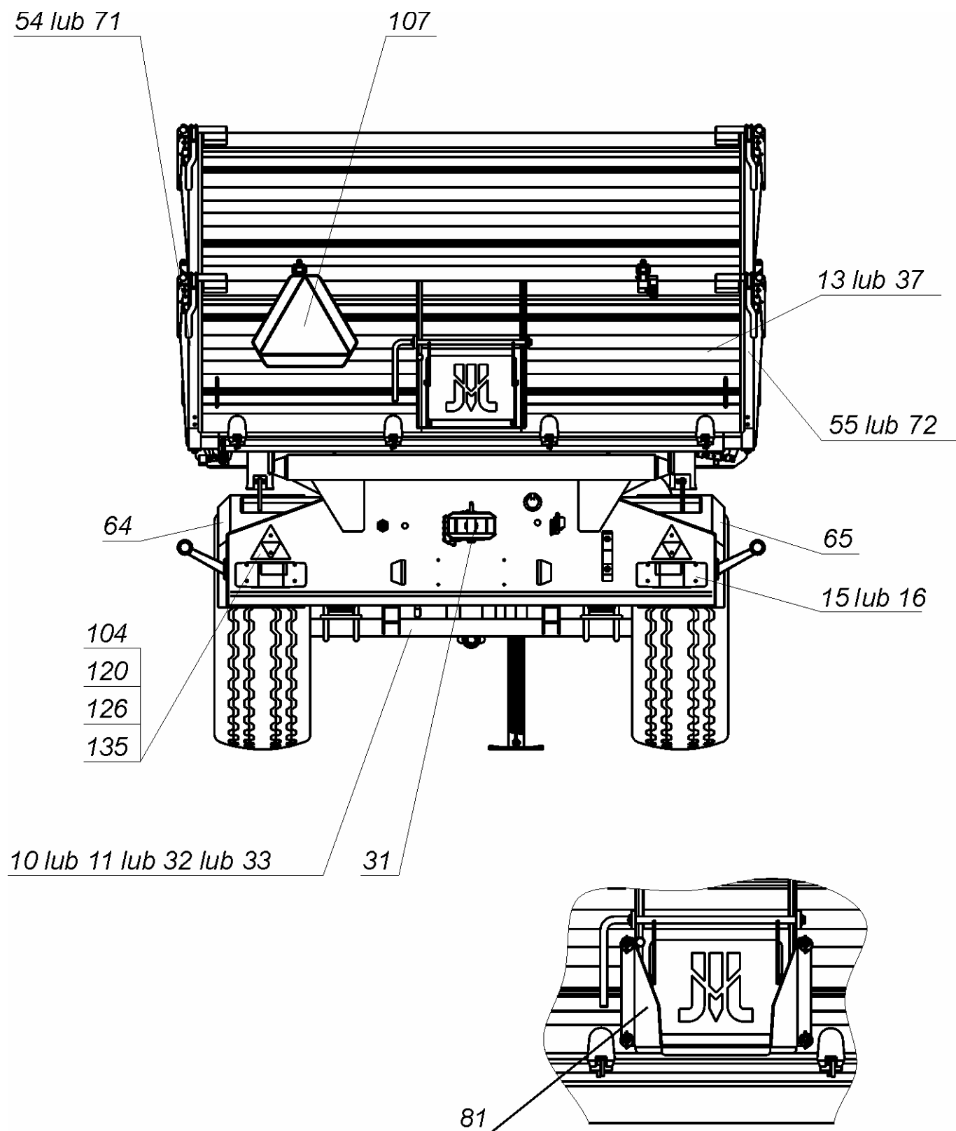
Rys. 17 Widok z tyłu
