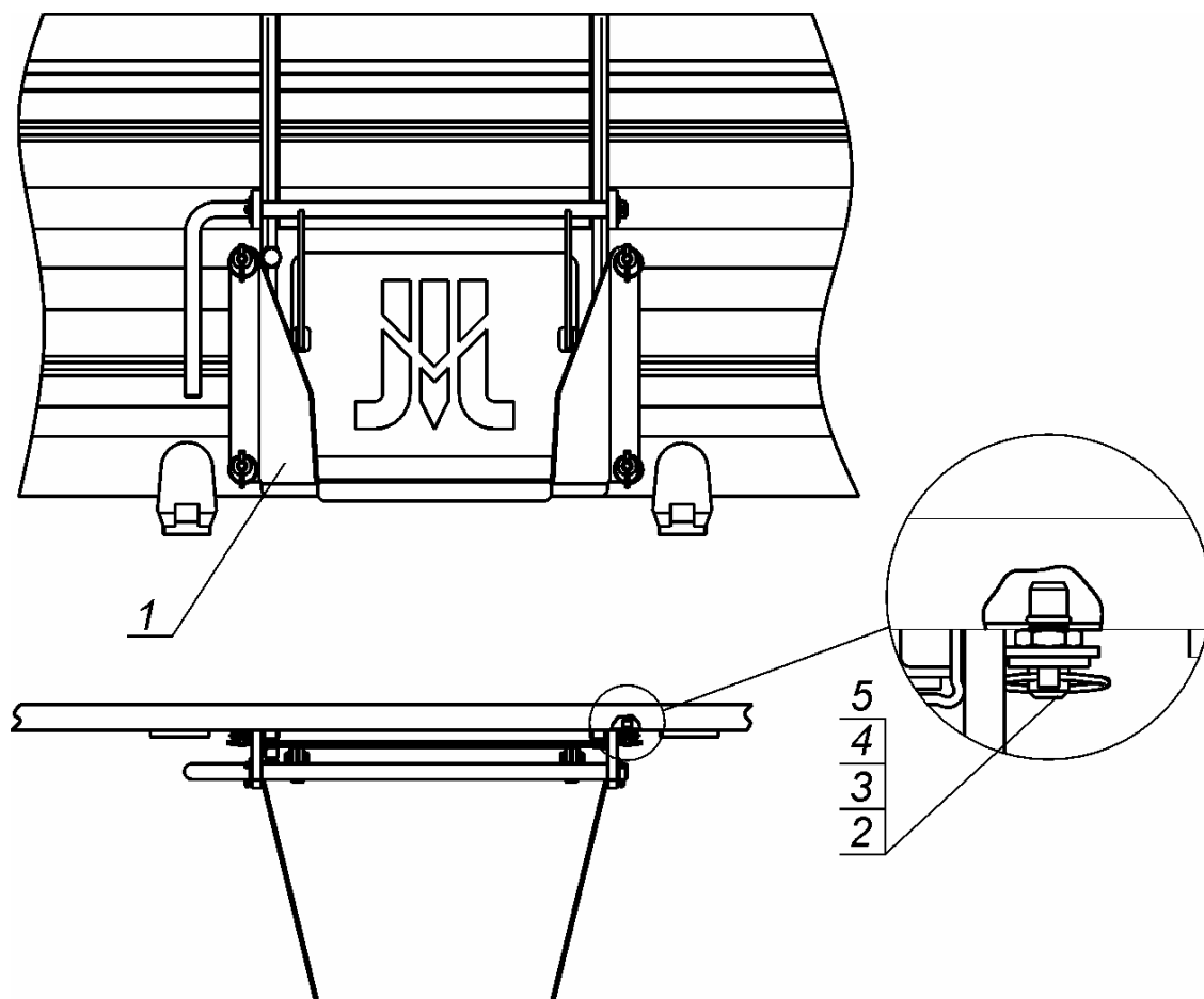
Rys. 46 Zsyp, kpl.
