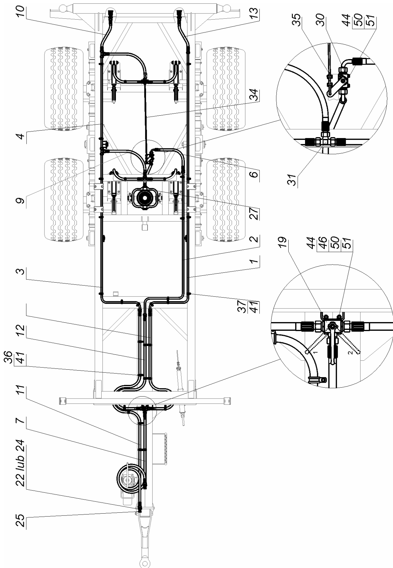
Rys. 27 Instalacja hydrauliczna, widok z góry
