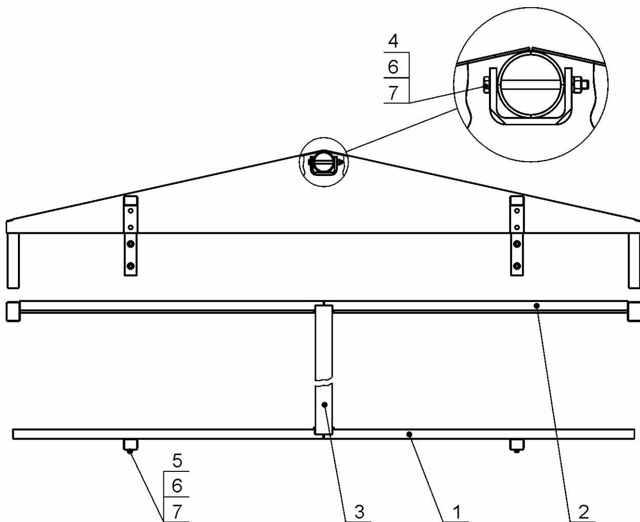
Rys. 50 Stelaż
