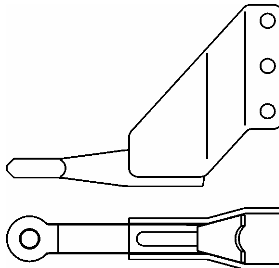
Rys. 37 Dyszel (Austria)
