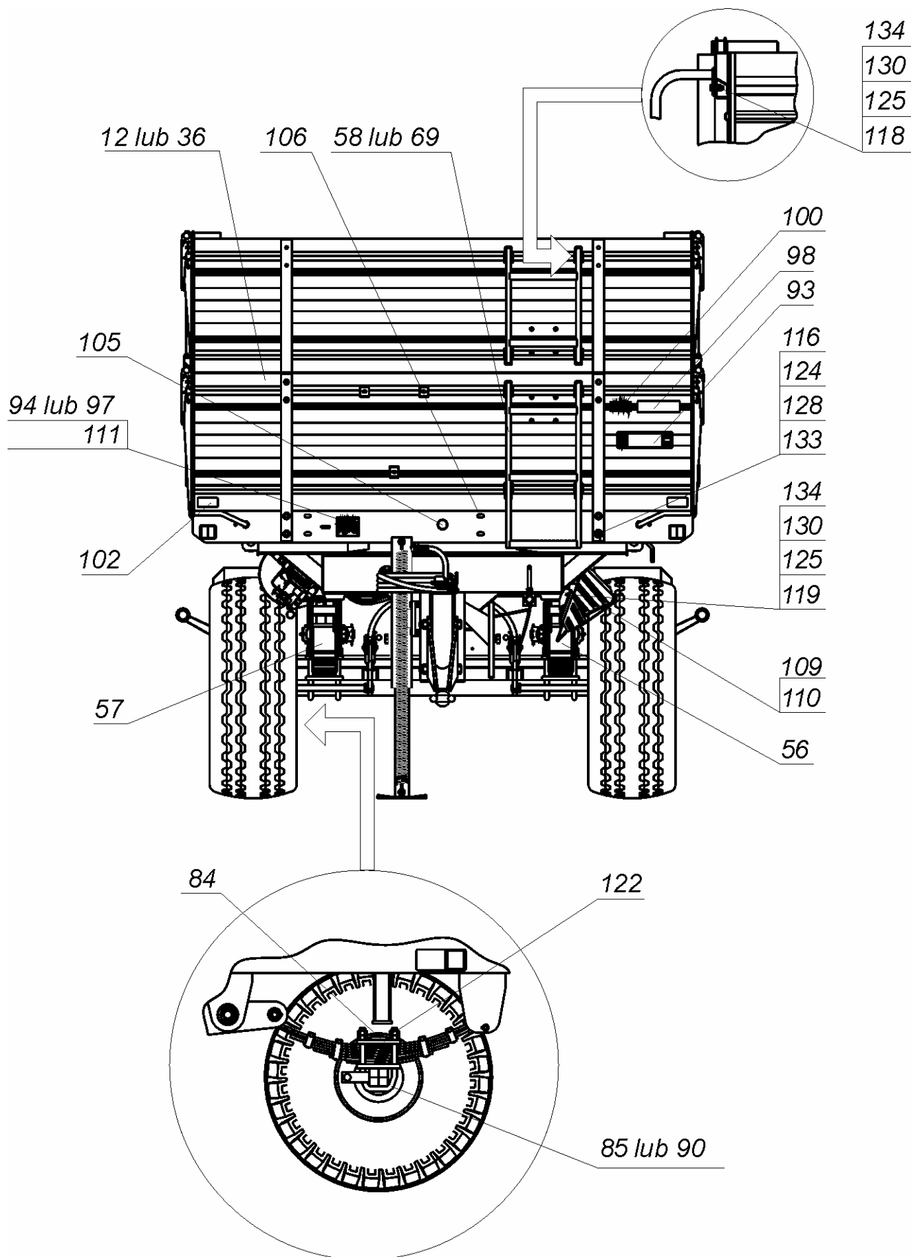
Rys. 16 Widok z przodu
