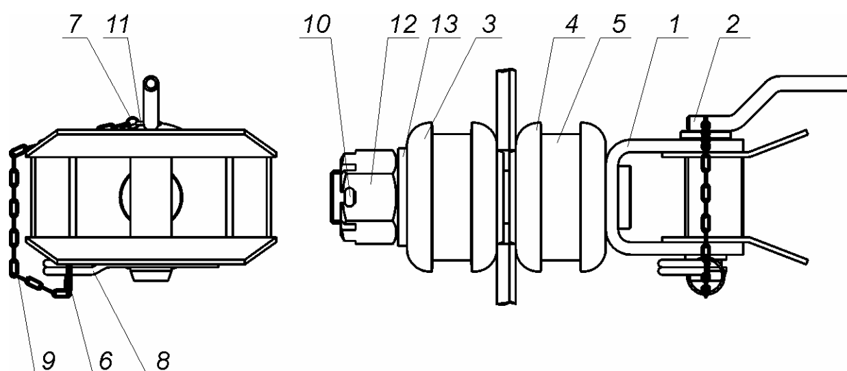
Rys. 38 Zaczep tylny
