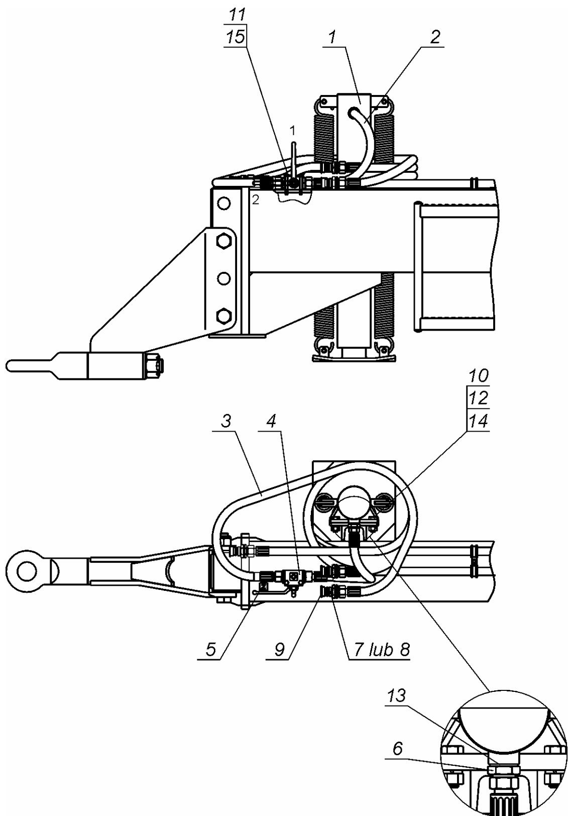
Rys. 32 Podpora hydrauliczna
