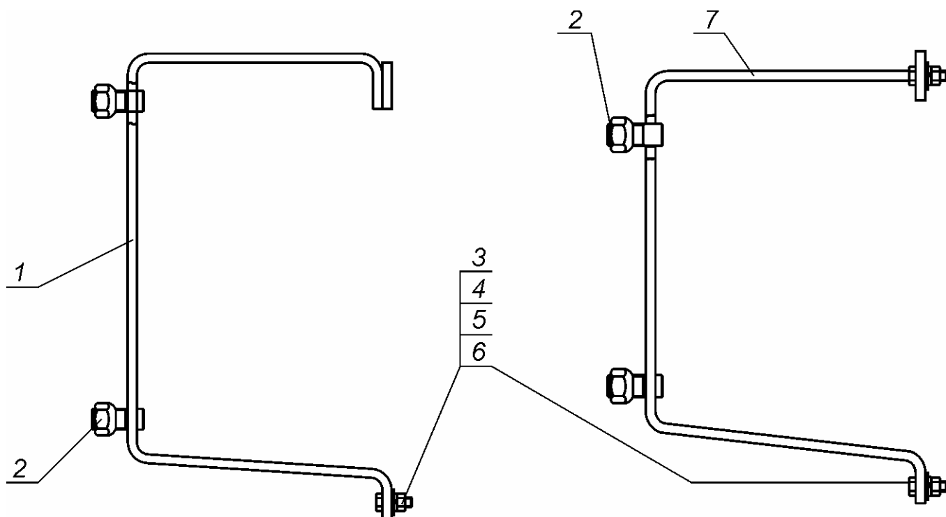
Rys. 49 Wieszaki koła zapasowego
