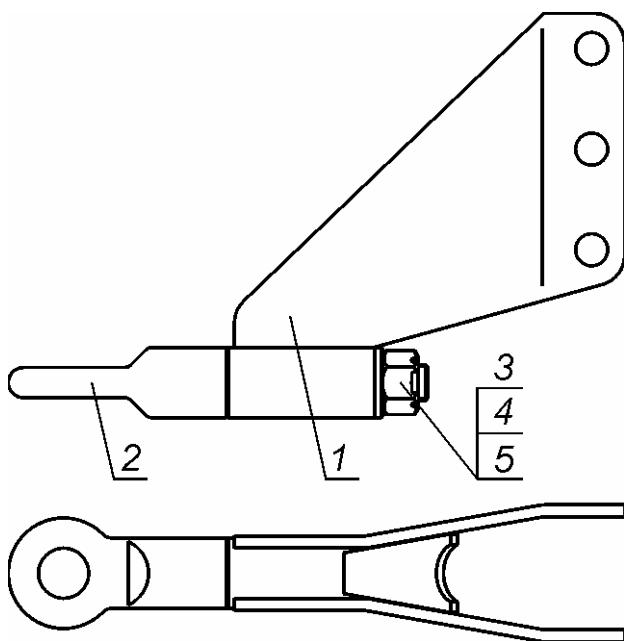
Rys. 34 Dyszel obrotowy
