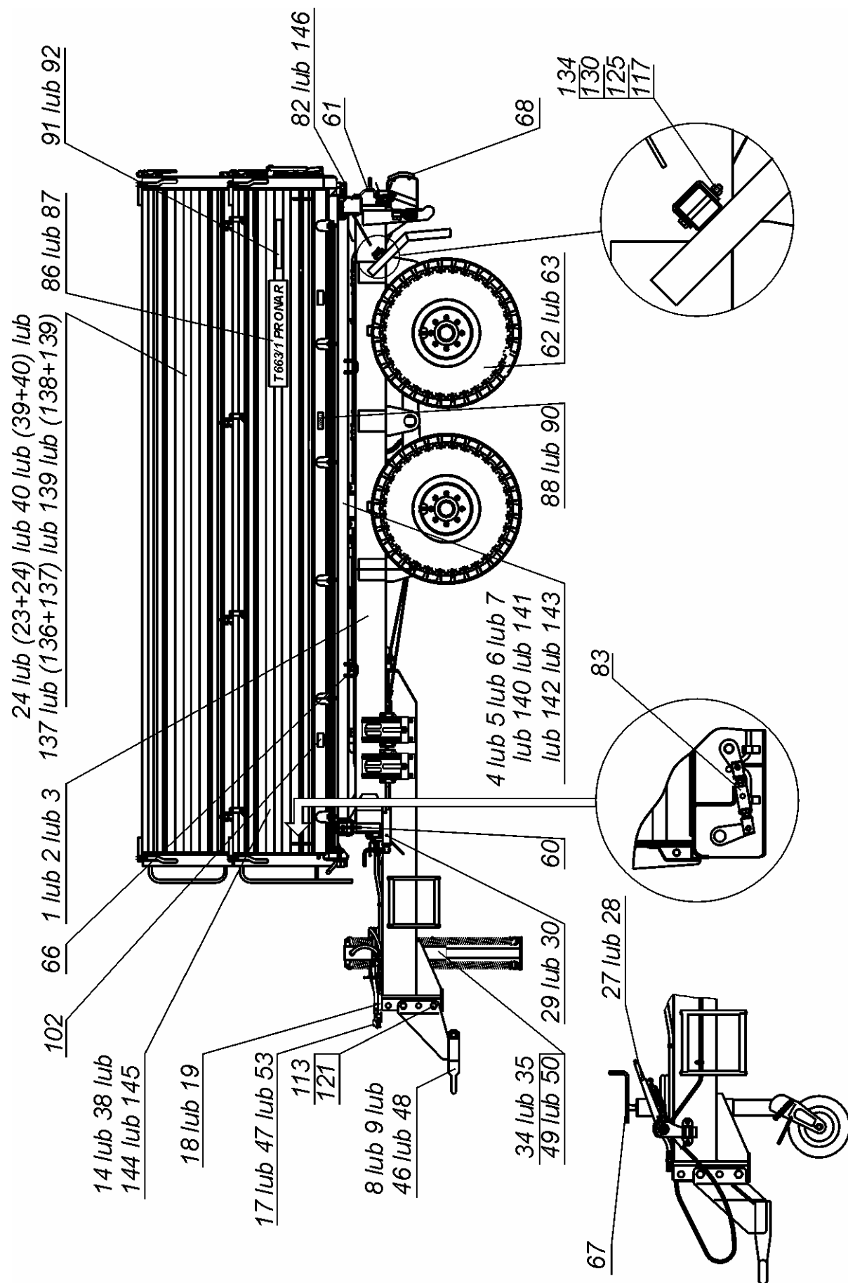
Rys. 18 Widok z boku
