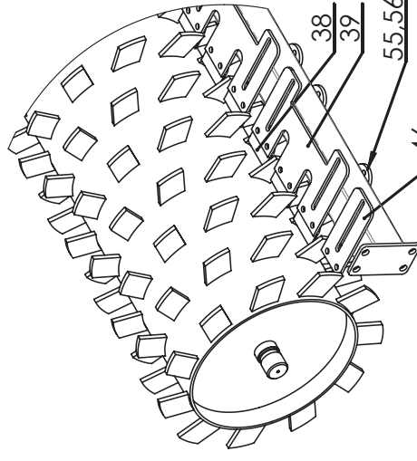
Wał Packer Ø460/550 Packer roller Ø460/550
