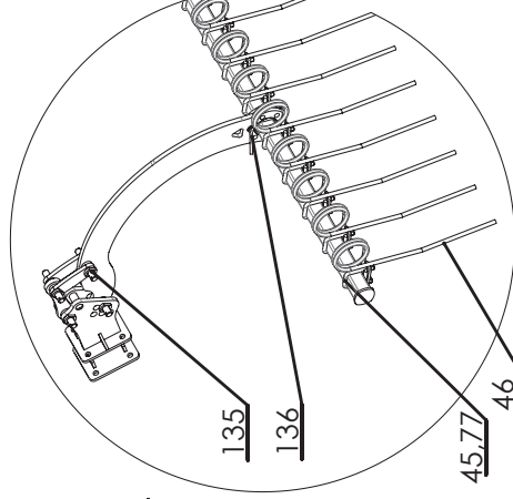
Wersja zawieszana Mounted version
