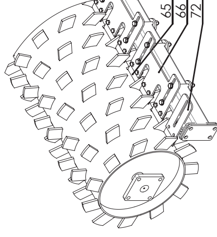
Wał Packer Ø460/550
