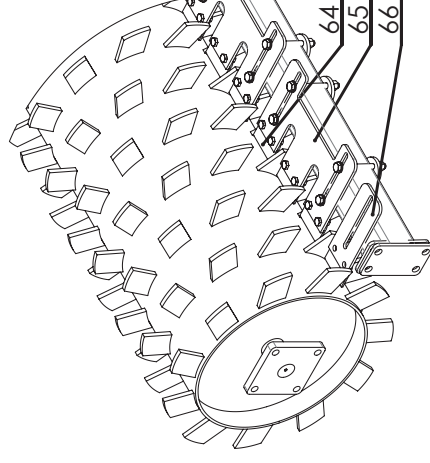
Wał gumowy Ø500 (nie pasujący dla wersji 3,0m) rubber roller Ø500 (doesn't fit 3m version)
