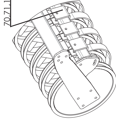
Wał U-ring Ø540 Wał T-ring Ø500 Ø600 U-ring roller Ø540 T-ring roller Ø500 Ø600
