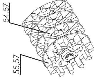
Wał U-ring Ø540 U-ring roller Ø540
