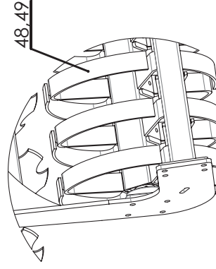
Wał gumowy Ø500 dla wersji 3,0m Rubber roller Ø500 for 3m version
