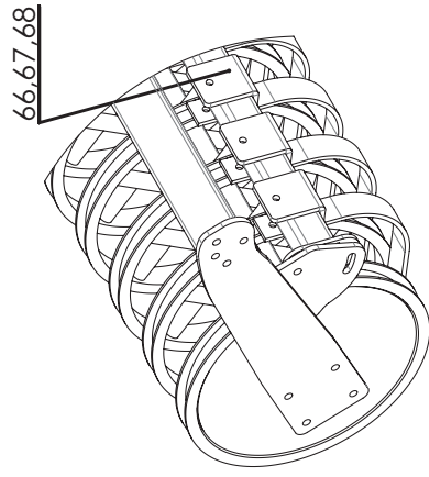
Wał U-ring Ø540 U-ring roller Ø540
