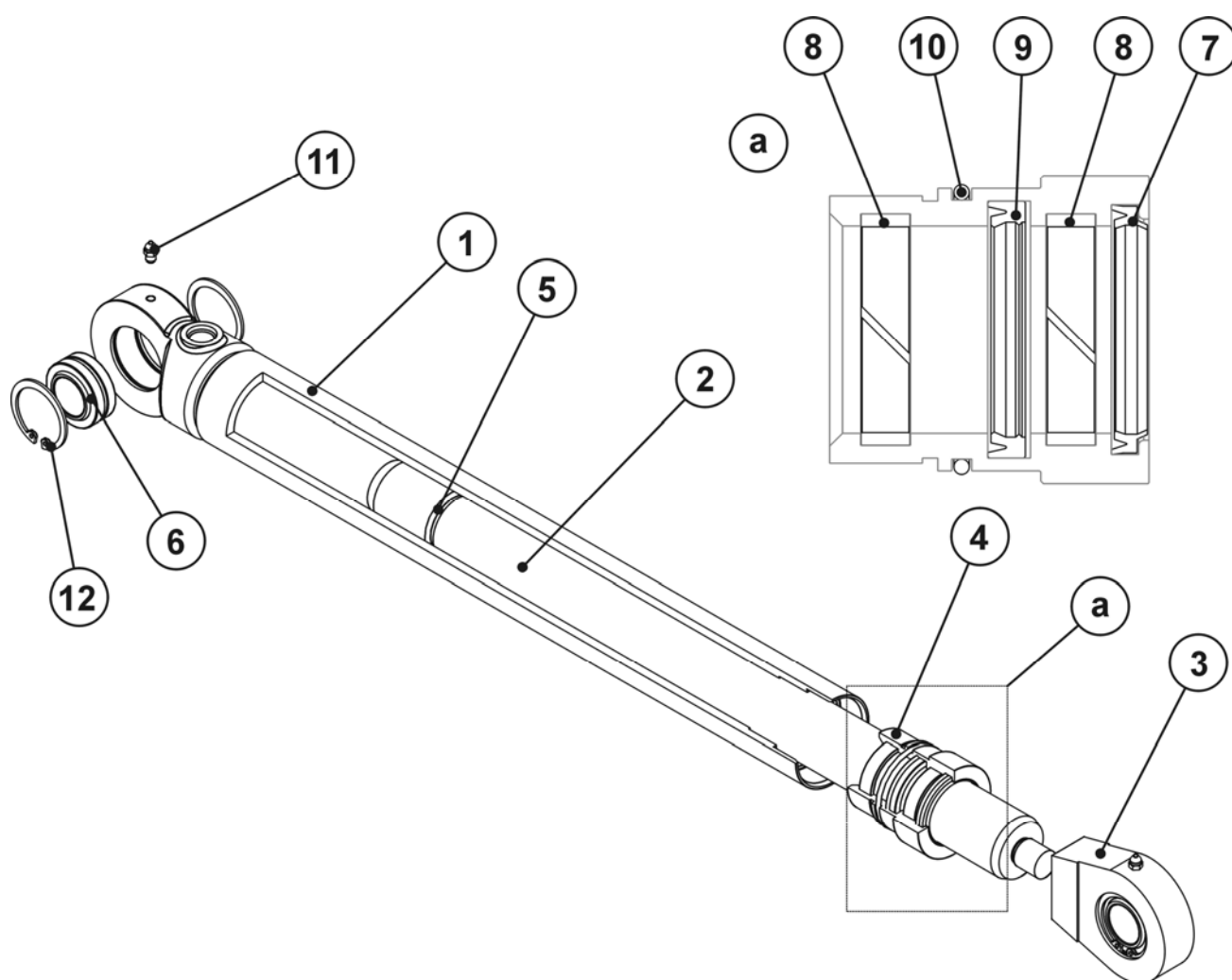
FIG. 34. PLUNGER CYLINDER 40/400
