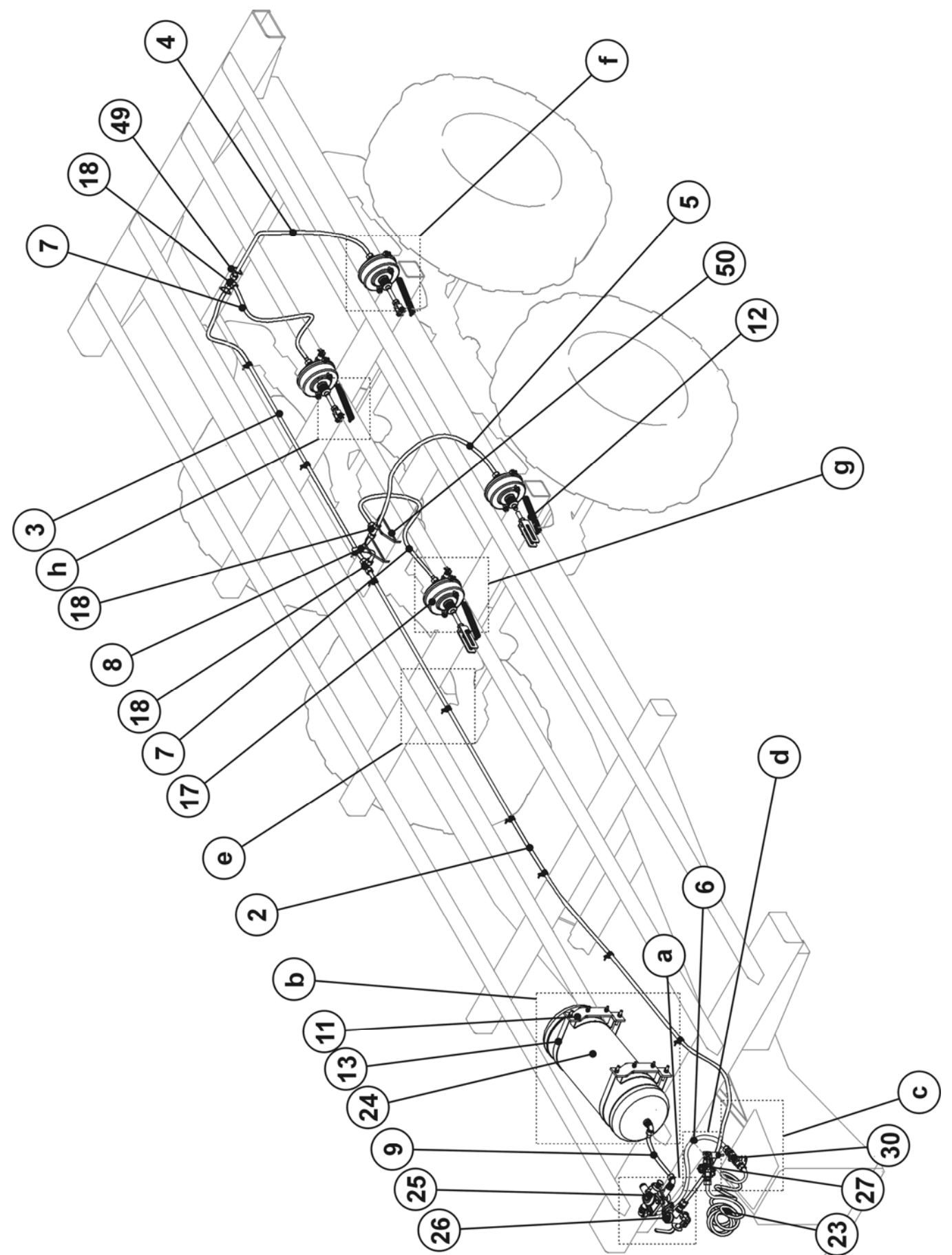
FIG. 39. SINGLE-CONDUIT PNEUMATIC SYSTEM
