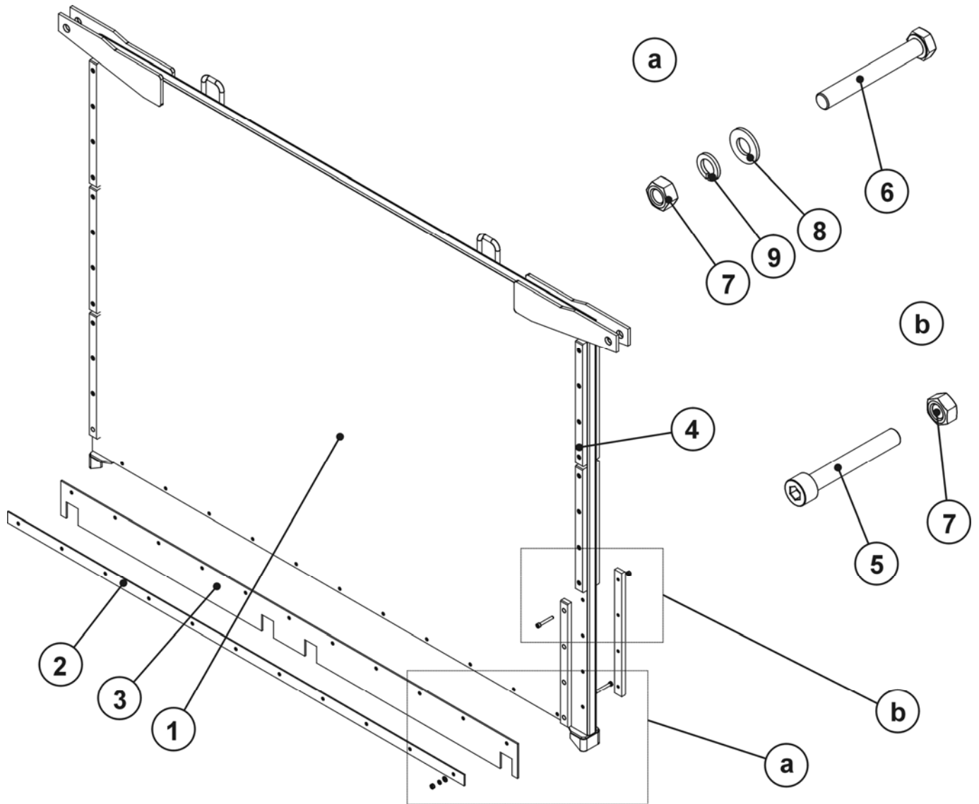
FIG. 13. GATE
