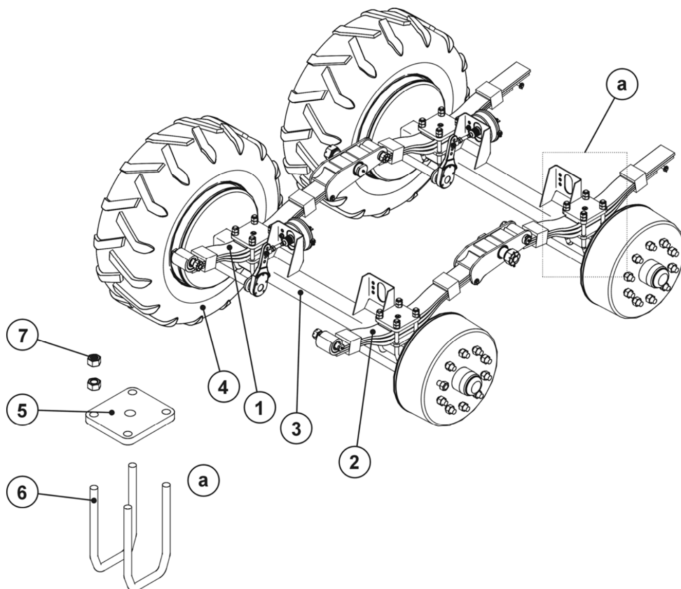
FIG. 26. SUSPENSION
