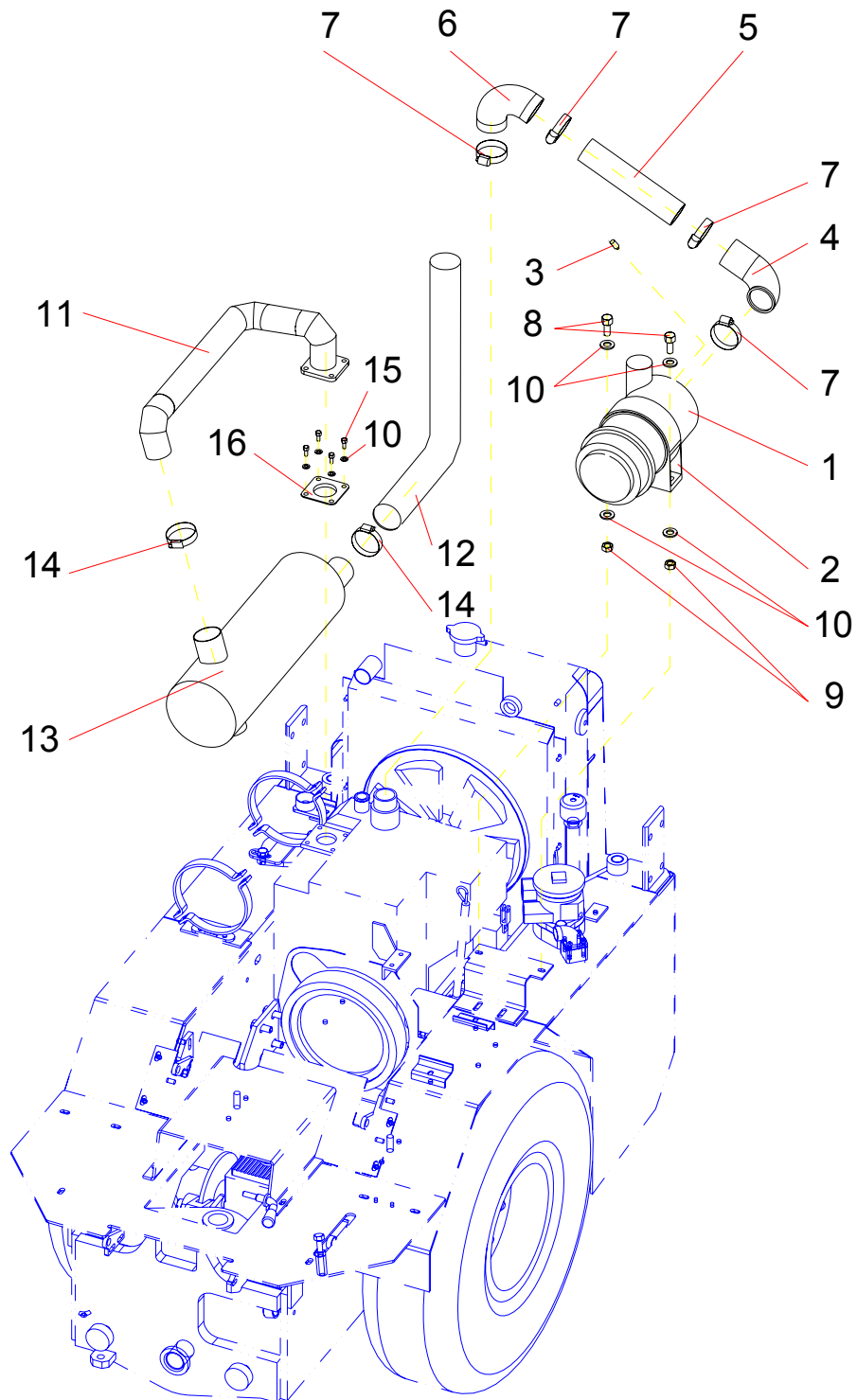
Fig.IV. LUFTFILTER - 2227.05.001 AUSPUFFANLAGE - 2227.06.002
