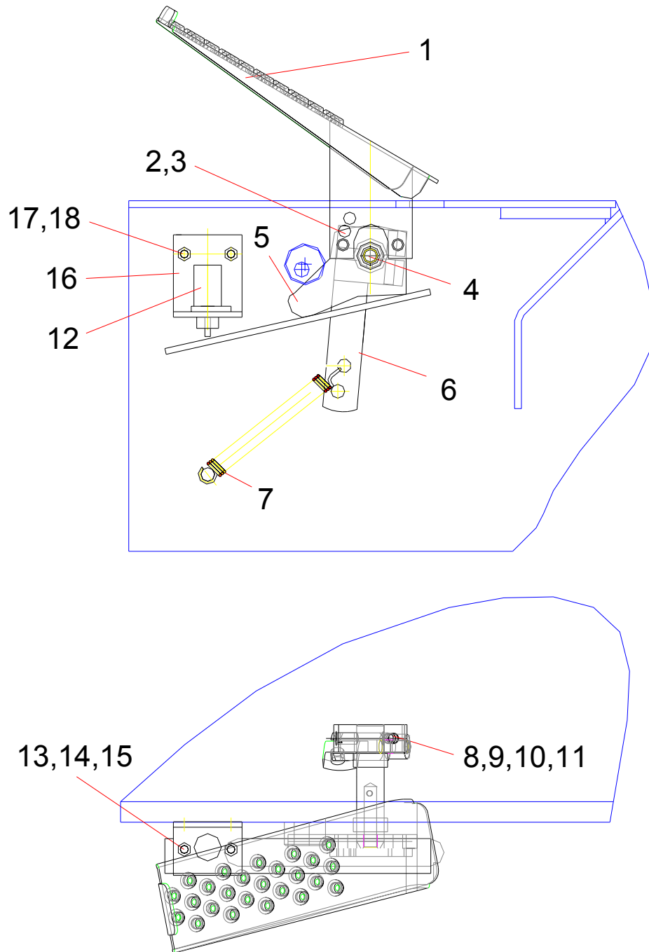
Fig.XV.A INCH-PEDAL - 2227.35.001.A
