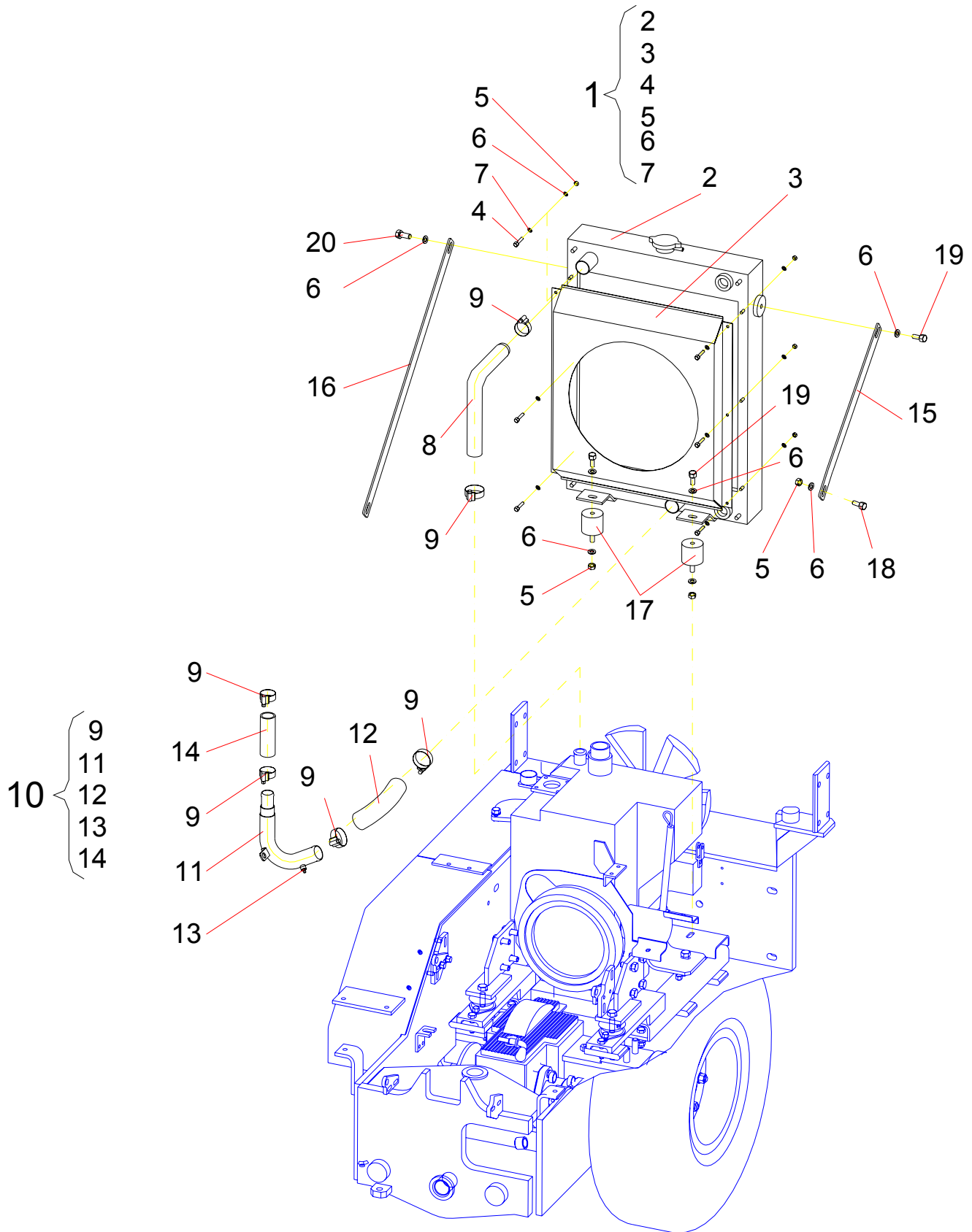
Fig.VII. KÜHLANLAGE - 2227.13.002
