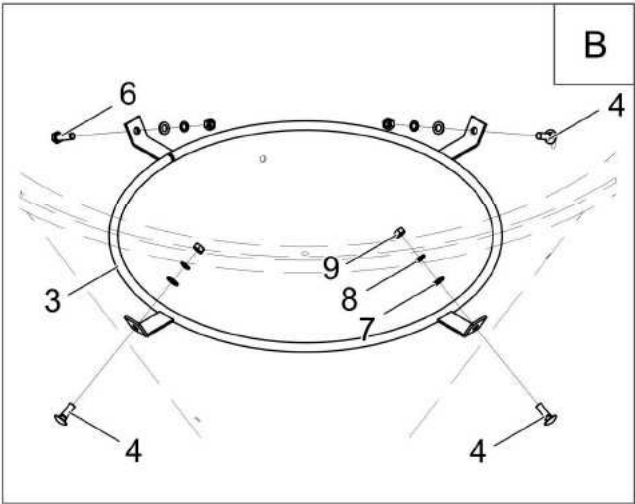
Sito i obręcz
