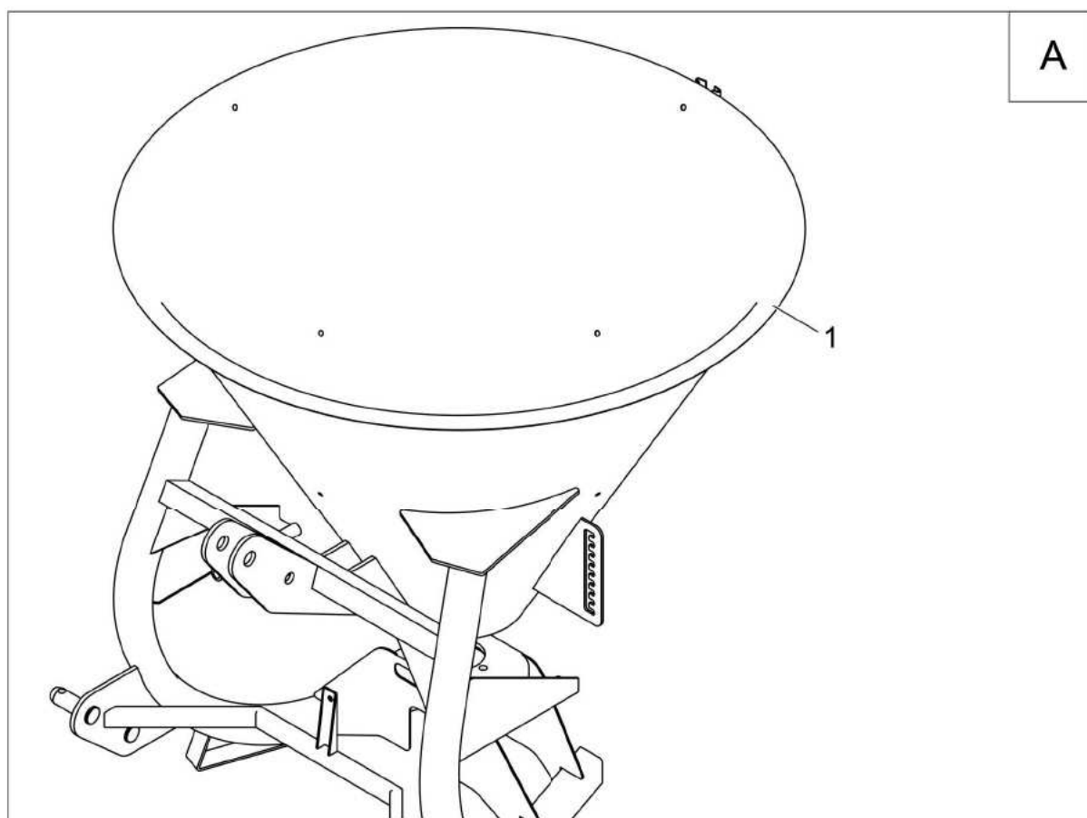
Konstrukcja nośna i kosz zasypowy
